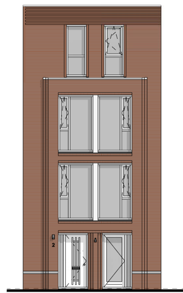
Voorgevel 1: 100
