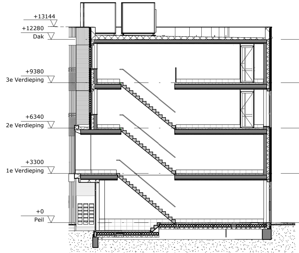
Doorsnede A
